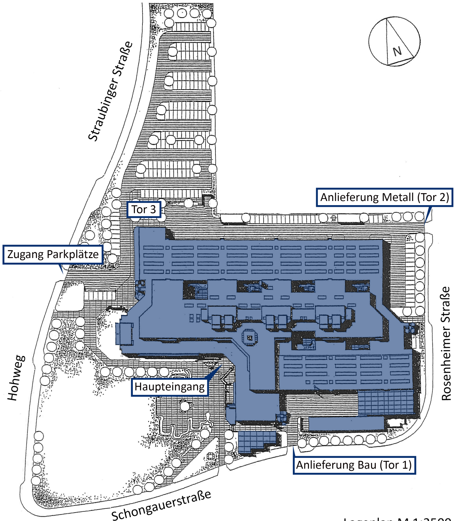
Lageplan M 1:2500
